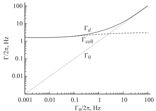
Рис. 3. Зависимость оптимальной столкновительной ширины линии \Gamma_{\text{coll}} и темновой ширины линии \Gamma_d от собственной ширины линии \Gamma_0 для калиевой кюветы диаметром 15 см.
