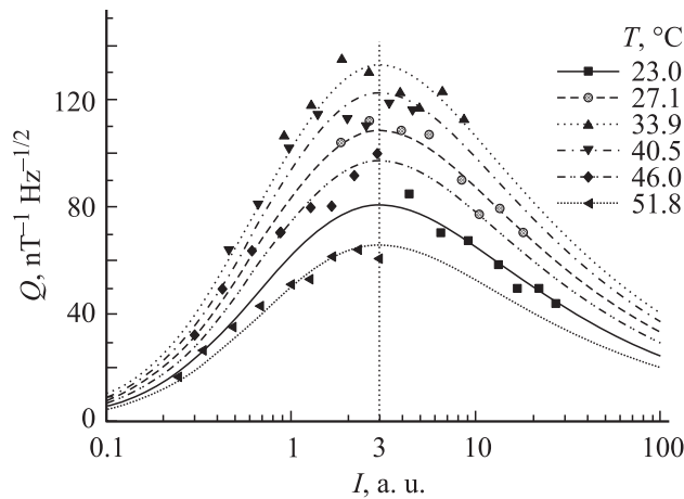
Рис. 6. Зависимость фактора качества в цезиевой ячейке от светового уширения при различных значениях температуры ячейки. Значки — эксперимент, линии — аппроксимация по формуле (16).
