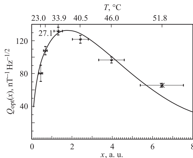
Рис. 7. Зависимость фактора качества в цезиевой ячейке от ее оптической толщины.
