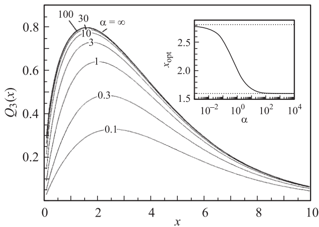
Рис. 2. Зависимость фактора качества Q от оптической толщины кюветы x при различных значениях \alpha . На врезке: зависимость оптимальной оптической толщины кюветы x_{\text{opt}} от \alpha .
